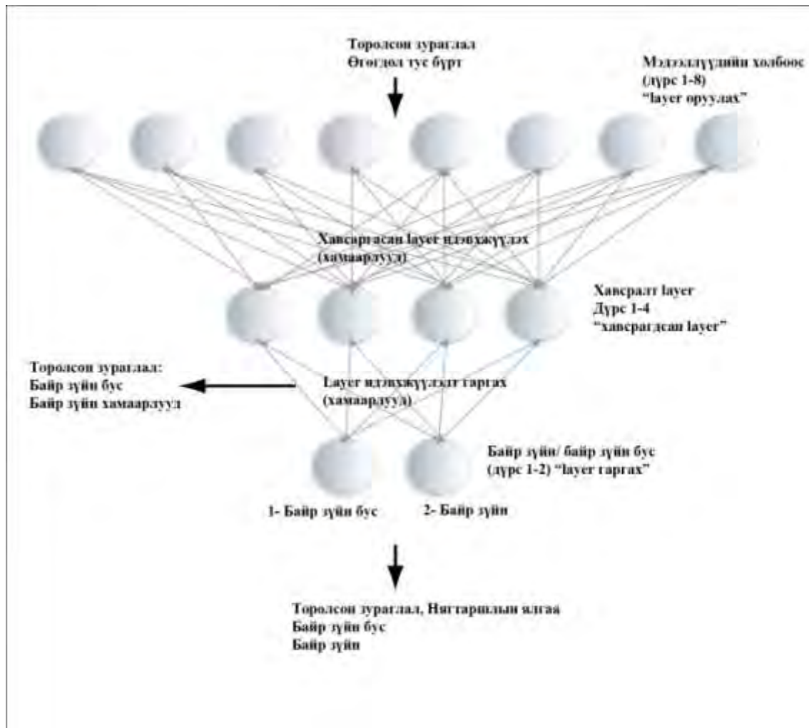
Зураг 14. Давхаргын бус болон гаралтын (гадаад) давхаргын зангилааг загварчилсан арга зүй
