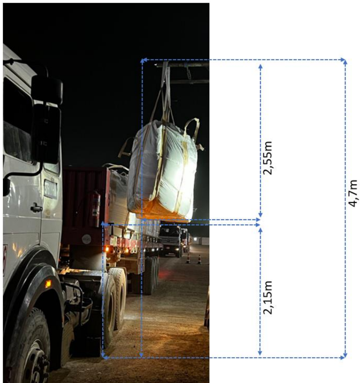
Зураг 02: Зэсийн баяжмалын уутыг өргөх одоогийн үйл явц ба ойролцоогоор өргөх өндөр.
