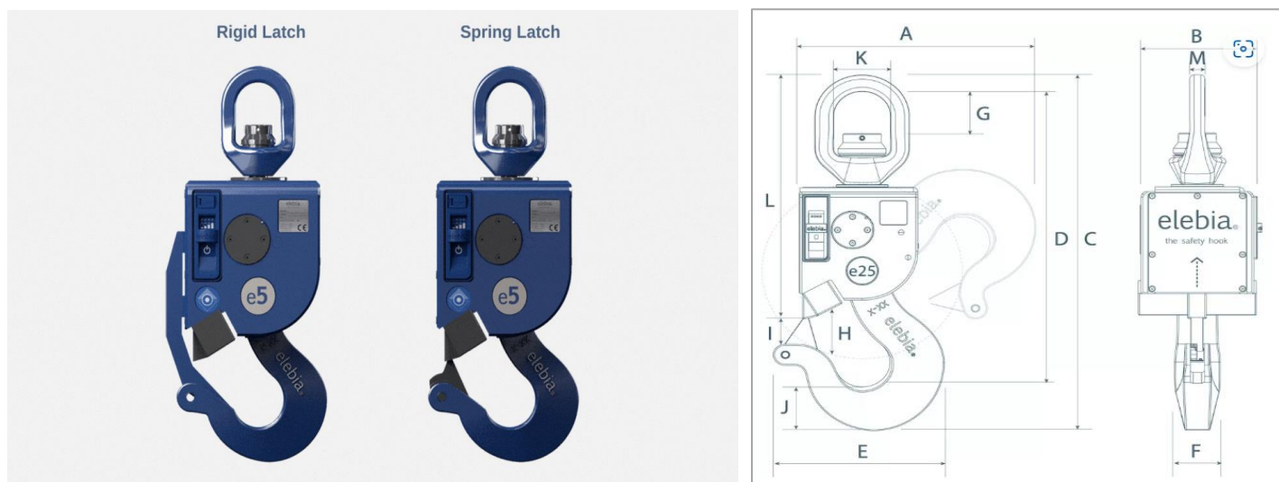
Зураг 04: Автомат дэгээ, зориулалтаар хийгдсэн тараагчийн хүрээтэй байх.
